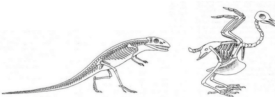
Figure 3. Transformation du squelette de théropode à celui d'un pigeon. Noter la compression antéro-postérieure du corps, la disparition de la queue et le positionnement du centre de gravité sous les ailes. [Source : Schéma de l'auteur]
