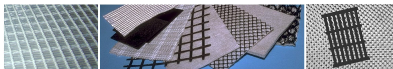
Figure 5. Exemples de géosynthétiques.
