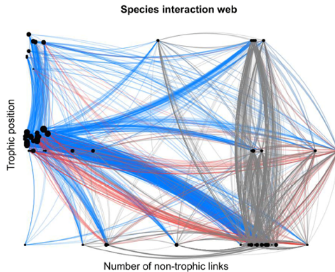
Figure 13. Représentation du réseau écologique d'interactions entre 106 espèces (figurées par les nœuds du réseau), appartenant à trois niveaux trophiques, composant une communauté marine intertidale au Chili. En bleu : interactions trophiques. En rouge et en gris : interactions non trophiques, respectivement positives et négatives. La diversité des interactions non trophiques augmente la résistance et la résilience du réseau. [Source : Kéfi et al., ref. [25], article sous licence Creative commons].
