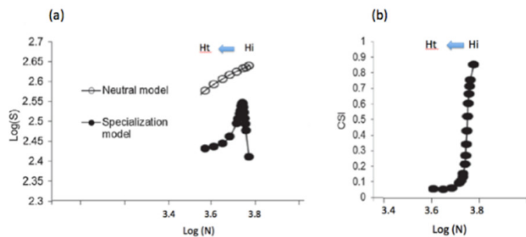
Figure 9. Simulation de l'impact de la transformation (dégradation) d'un habitat, avec réduction progressive de sa capacité de charge, sur une méta-communauté alimentée par un pool régional de 500 espèces. H_i : habitat initial, H_t : habitat transformé, de moindre capacité de charge pour la communauté considérée ( K_t < K_i ). (a), relation à l'équilibre entre la richesse spécifique (nombre d'espèces S ) et l'abondance (nombre d'individus N ) de cette communauté selon le modèle utilisé, en coordonnées logarithmiques. Courbe du haut (en blanc) : modèle stochastique neutre : les 500 espèces sont toutes équivalentes sur le plan démographique (i.e., mêmes probabilités de colonisation, reproduction et survie locale par individu). (b), Relation à l'équilibre entre l'indice de spécialisation (CSI) de cette communauté et le logarithme de son abondance ( \log N ), selon le modèle de spécialisation. [Schémas A. Teyssède, adapté de Teyssède et Robert ref. [18]. Reproduit de 'Regard sur la biodiversité' (R103), sous licence Creative commons]
