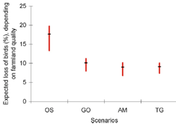
Figure 5. Estimation de l'impact de l'agriculture sur l'abondance de l'avifaune mondiale (en nombre d'individus) attendu pour la période 1990-2050, selon le scénario socioéconomique (et d'usage des terres) du MEA. Les barres verticales rouges représentent les intervalles de confiance ( p > 0,95 ) autour des valeurs calculées pour les quatre scénarios, selon l'usage des terres estimé par le MEA. OS : Order from Strength (scénario réactif et régional) ; GO : Global Orchestration (proactif, coordonné à l'échelle mondiale) ; AM : Adapting Mosaic (proactif, régional) ; TG : Technogarden (réactif, coordonné entre régions). [Source : Adapté de Teyssèdre et Couvet, ref. [7]. Reproduit de 'Regard sur la biodiversité' (R103), sous licence Creative commons].
