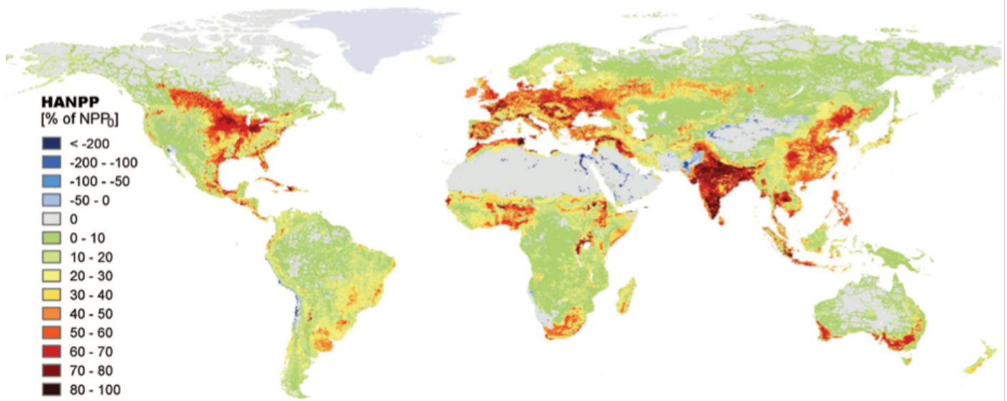
Figure 3. Représentation géographique de l'appropriation de la production primaire nette par les humains (HANPP), en tant que pourcentage de la production primaire nette potentielle locale (NPP 0 ). De l'ordre de 10% en Asie centrale et en Australie, cette proportion s'élève à près de 60% en Asie du Sud et environ 45% en Europe de l'Est et du Sud-Est [NB : Les taches bleues correspondent aux régions où la production primaire est accrue par les activités humaines, principalement via l'irrigation. [Source : Haberl et al., [2], © National Academy of Sciences. Reproduit de 'Regard sur la biodiversité' (R103), sous licence Creative commons.]
