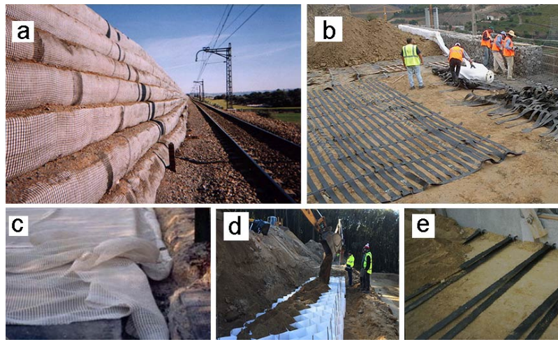
Figure 2. Renforcement des massifs de soutènement. (a) Mur renforcé par géosynthétiques ; (b) renforcement par géogrilles ; (c) Renforcement par nappes géotextiles ; (d) Renforcement par structures alvéolaires (procédé Armater [1]) et (e) renforcement par bandes géotextiles.
