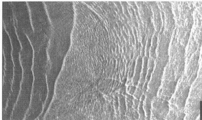
Figure 2. Image satellite des ondes internes obtenue par radar à synthèse d'ouverture (SAR). Elle montre la convergence/divergence des ondulations dans la mer d'Andaman. [Source: Osborne AR & Burch TL.1980, ref [2], Droits réservés].
