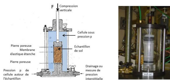
Figure 4. L'essai triaxial permet de caractériser la rigidité et la résistance d'un sol situé en profondeur. A gauche, principe de l'essai (métrologie non représentée). A droite, photo d'une cellule triaxiale. L'échantillon cylindrique est soumis à une contrainte de confinement p (simulant la profondeur), puis comprimé (force axiale F représentant l'action d'un ouvrage proche), des petites déformations jusqu'à la rupture. [source : Marc Boulon]
