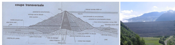
Figure 3. Le barrage en terre et enrochements de Grand-Maison, sur l'Eau d'Olle, dans les Alpes, mis en service en 1988. Un des grands barrages du monde, hauteur 140 m, longueur en crête 550 m. Ci-dessus coupe montrant le noyau (argileux d'étanchéité), le rideau d'étanchéité dans le lit de la rivière, complétant l'étanchéité, les recharges en enrochements, amont et aval, assurant la stabilité. A droite, photo du barrage et du réservoir, vus de l'aval. Ce barrage est la partie supérieure d'une STEP (station de transfert d'énergie par pompage, 1820 MW, 300 Gwh/an), permettant de stocker sous forme hydraulique l'énergie électrique non utilisée aux heures creuses. [Source : Gauche, Comité français des barrages et réservoirs, 2012, Technologie des barrages ; Droite, By Douchet Quentin [GFDL ( http://www.gnu.org/copyleft/fdl.html ) or CC BY-SA 3.0 ( http://creativecommons.org/licenses/by-sa/3.0/ )], via Wikimedia Commons]
