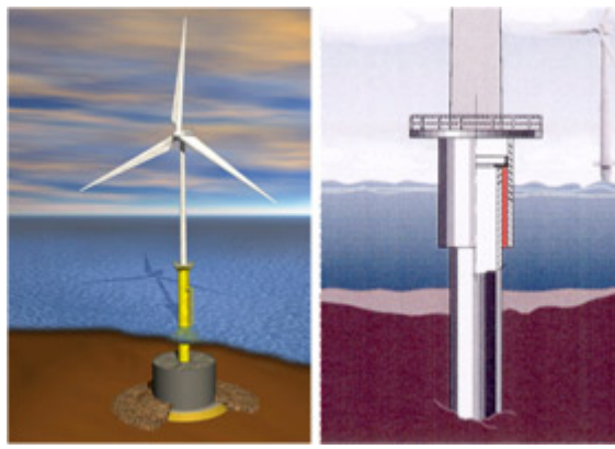
Figure 1. Éoliennes off-shore 5 MW, 30 m d'eau, 110 m émergés, à gauche embase poids de diamètre 30 m, sur sols rocheux durs (granite) ; à droite fondation sur monopile battu et/ou foré de diamètre 6 m, sur sols rocheux tendres (craie). [source : A. Puech, 2008, Cours de géotechnique marine, ENSHMG ]
