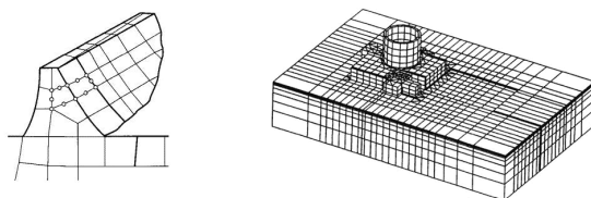
Figure 5. Maillage de 2 ouvrages en éléments finis. A gauche, un barrage (très simplifié) et sa vallée. A droite une centrale et son site proche. La méthode consiste à écrire l'équilibre mutuel et les déformations d'un grand nombre de petits éléments de volume, formés de matériaux possédant chacun leur rigidité et leur résistance. [source : MESTAT, P., (1997), Maillages d'éléments finis, conseils et recommandations, BLPC 212, 39-64]
